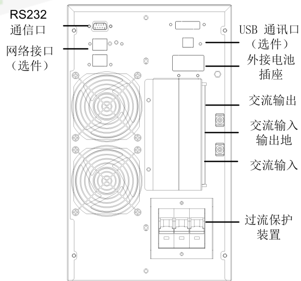
3C10KS 后面板
