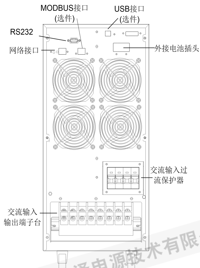
3C15K(S)/20K(S)后面板
