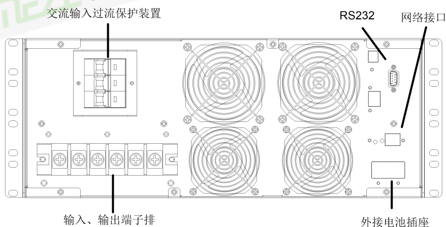
3C15KRS/20KRS 机架式 UPS 后面板示意图
