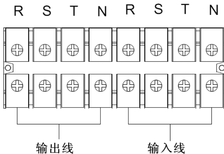
HV 30K(L)/40K(L) and LV 15K(L)/20K(L)端子排示意图
