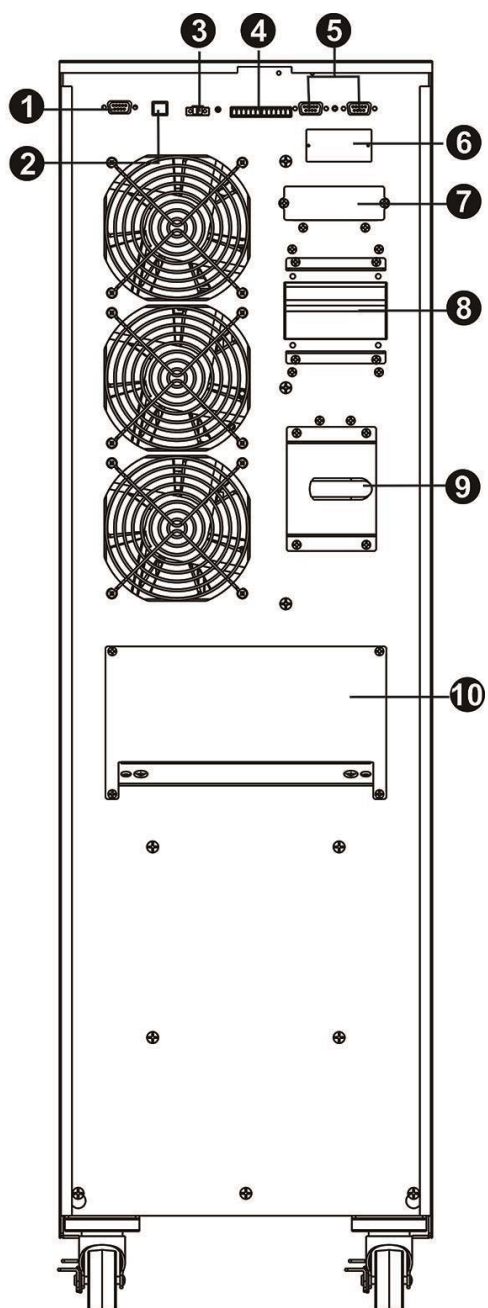
图 2: HV 40K(L)/LV 20K(L)背板
