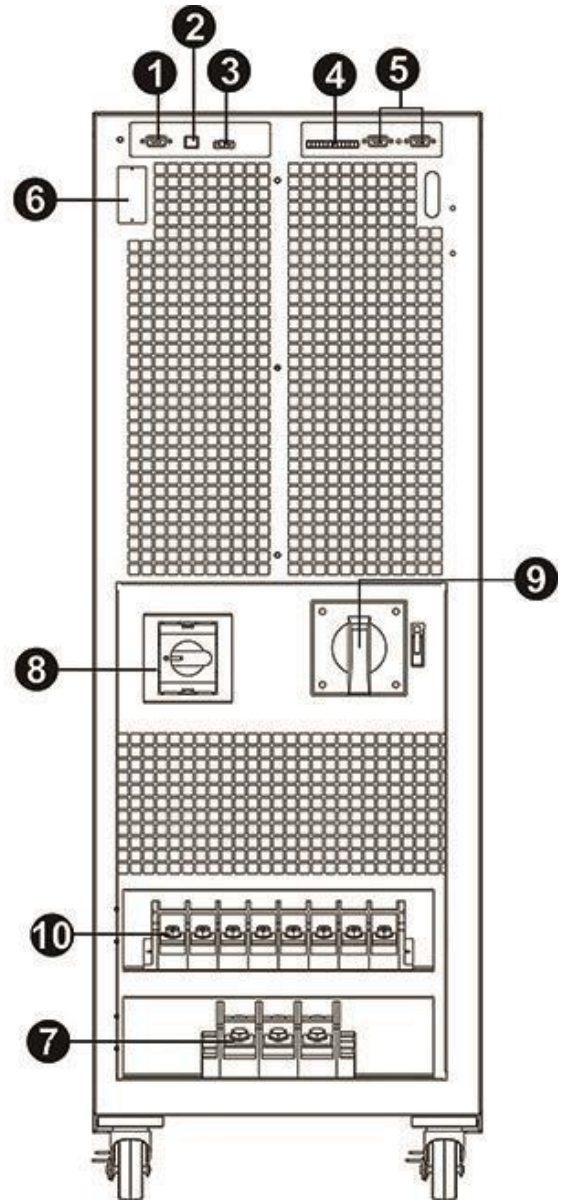
图 5: HV 80KL/LV 40KL 打开来前面板视图
