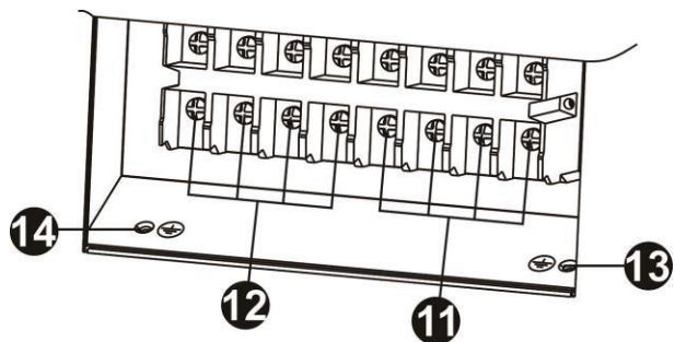
图 3: HV 30K(L)/LV 15K(L)/ HV 40K(L)/LV 20K(L) 输入/输出端子
