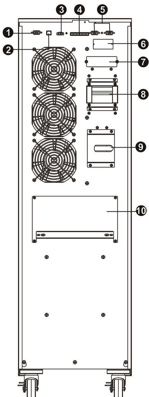
图 1: HV 30K(L)/LV 15K(L)背板
