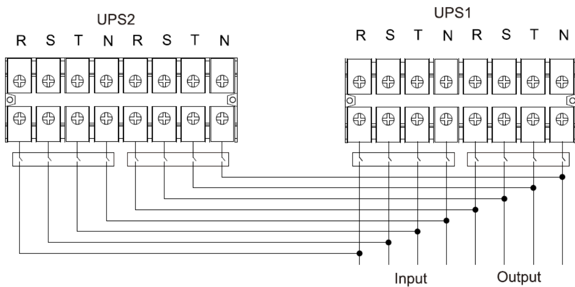
HV 60KL/80KL and LV 30KL/40KL 并机系统接线图
