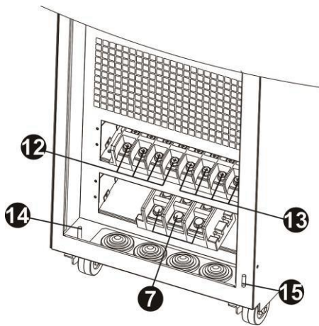
图 4: HV 60KL/LV 30KL 打开来前面板视图
