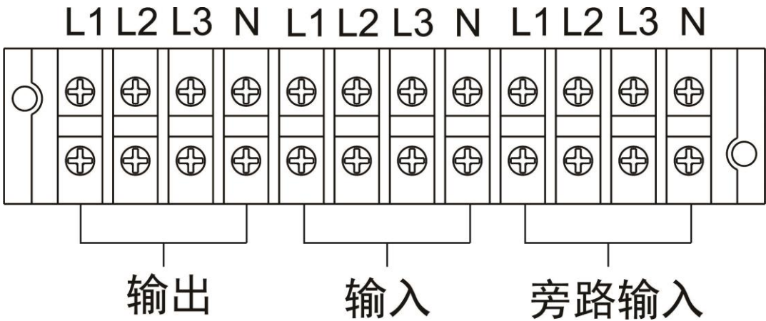
10K（L），20K（L）端子布线图
