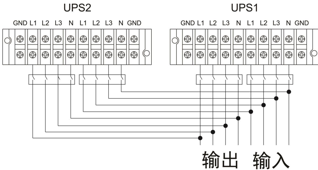
30K(L)并联系统布线图
