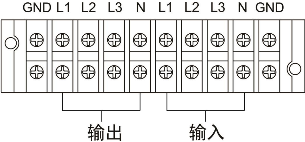
30K（L）端子布线图
