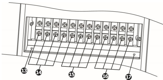
图 4: 10K(L)/15K(L)/20K(L) 输入/输出端子台
