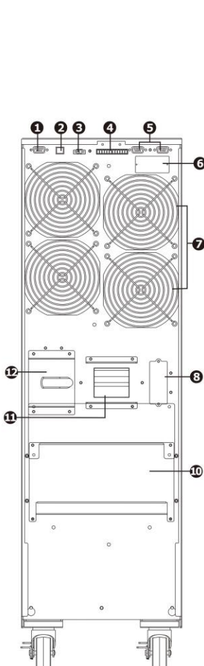
图 1: 10K(L)/15K(L)/20K(L)背板图
