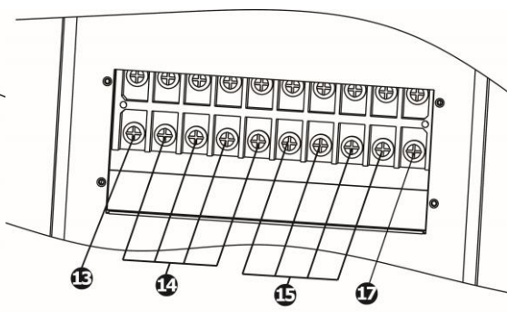
图 5: 30K(L) 输入/输出端子台
