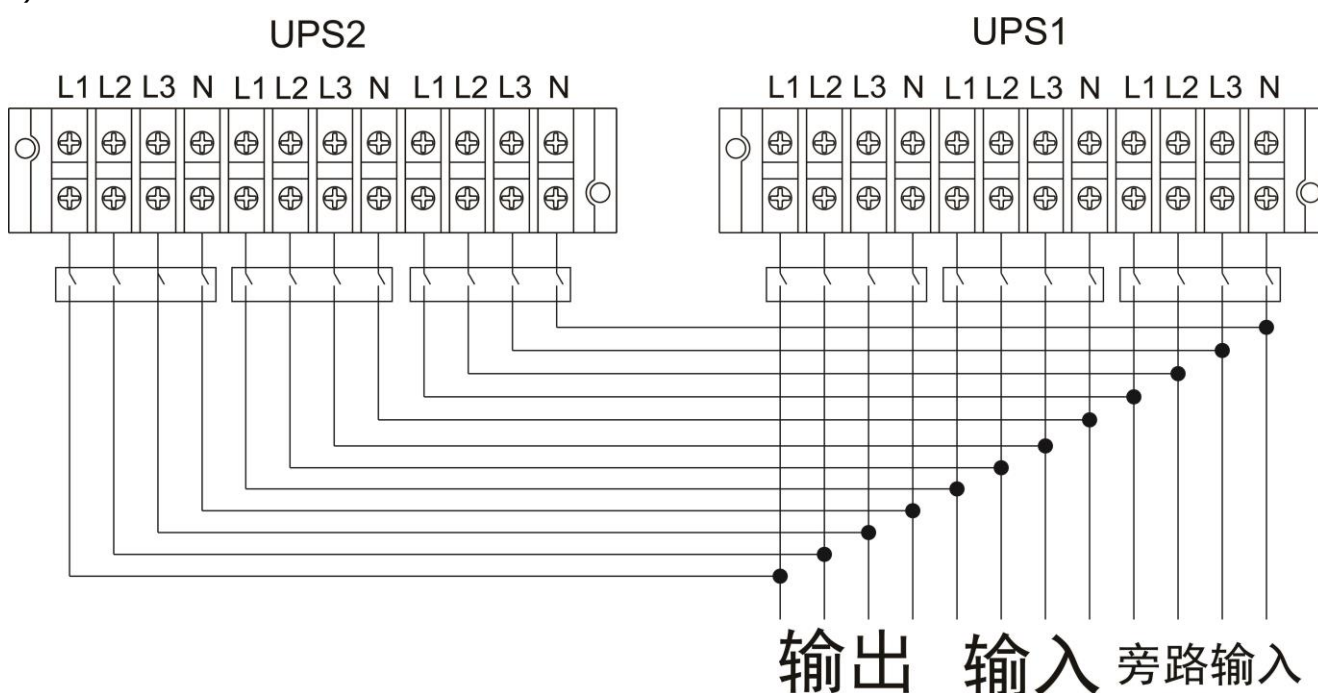
10K (L) ,20K(L)并联系统布线图
