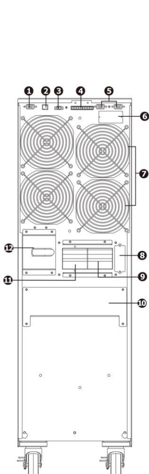
图 1: 10K(L)/15K(L)/20K(L)背板图
